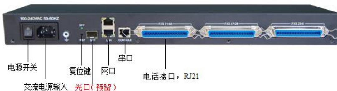
后面板图
