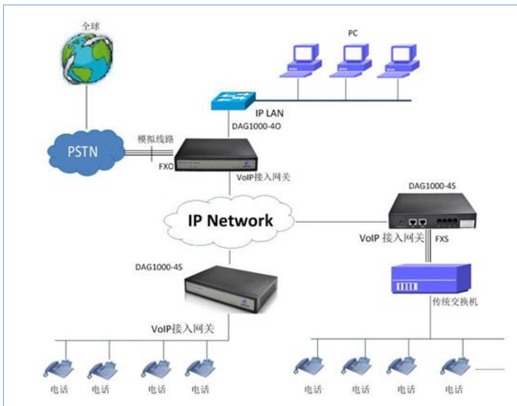
应用拓扑图
